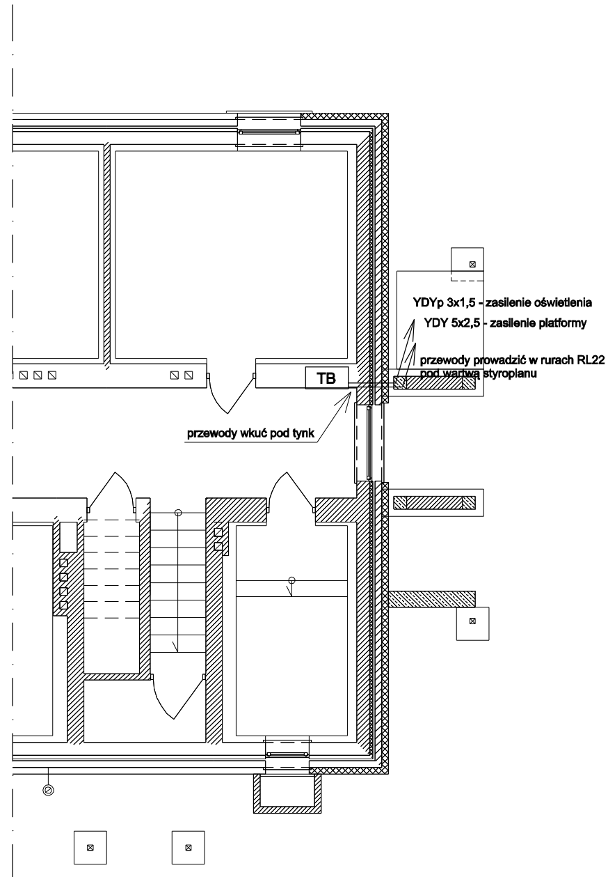
RZUT PIWNICY
