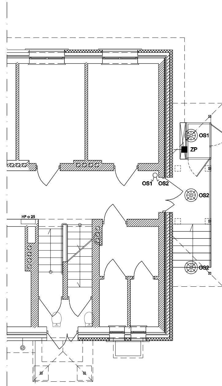
RZUT PARTERU
