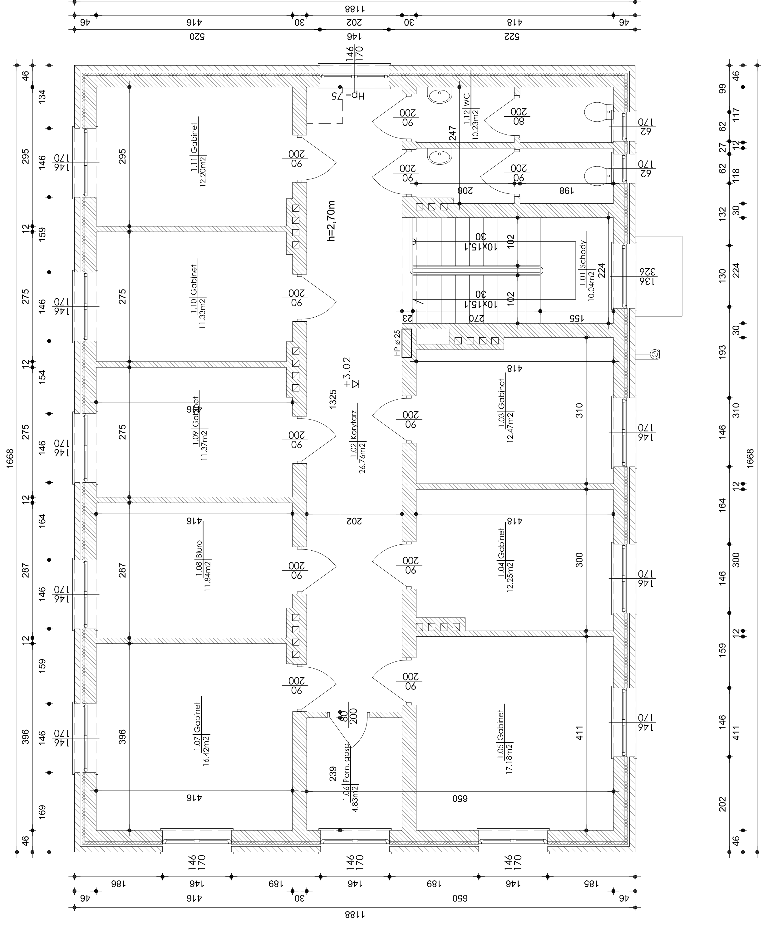
RZUT PIĘTRA 1:50
