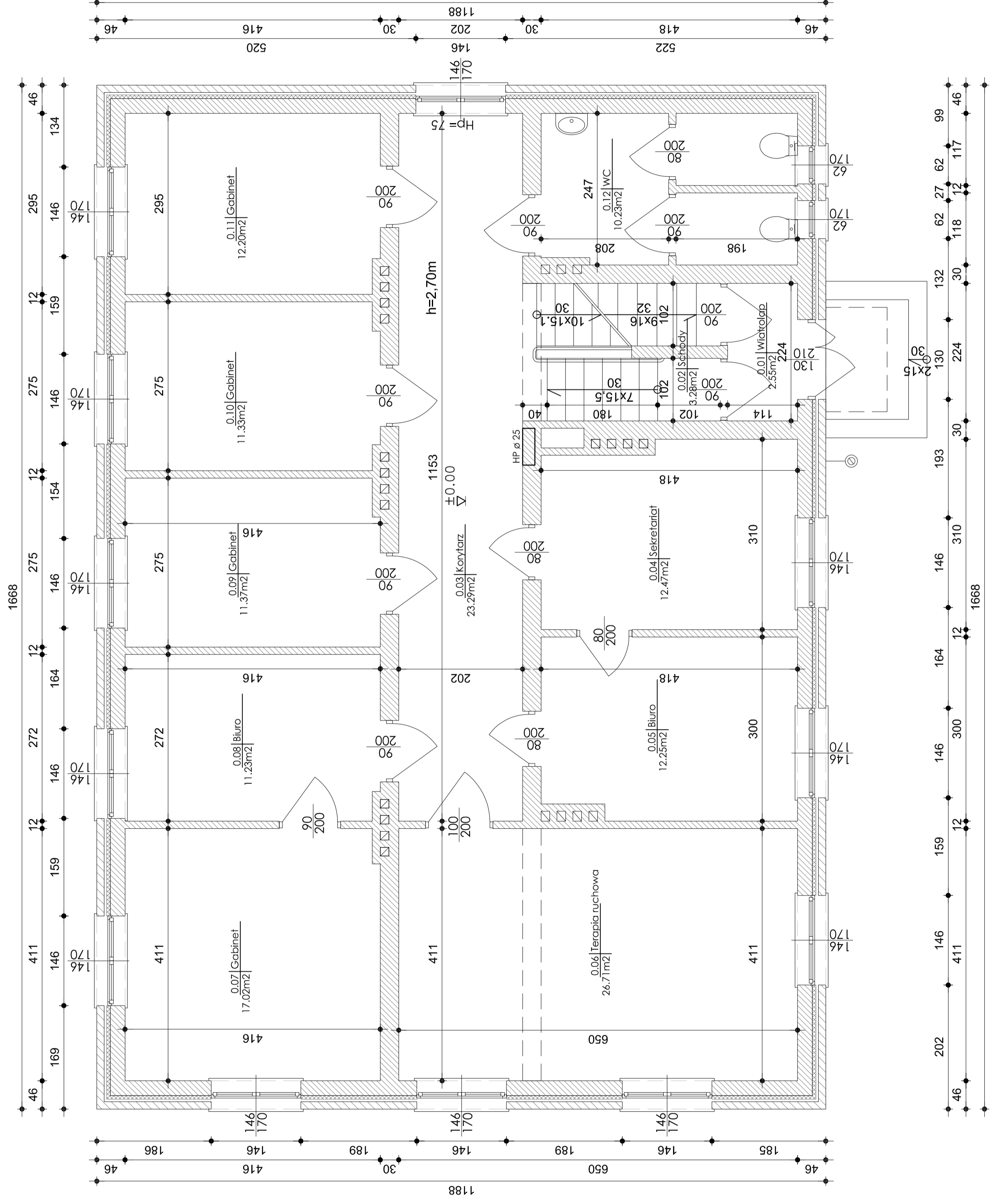
RZUT PARTERU 1:50
